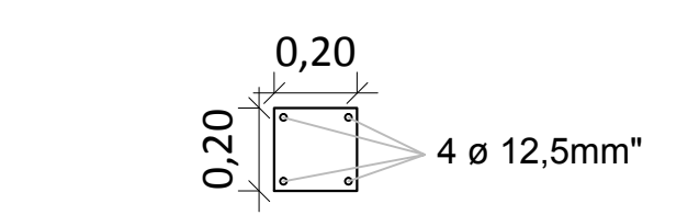
DETALHE PILAR ESCALA 1:20
