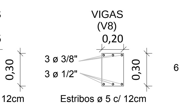
VIGAS (V8) 0,20 0,30 3 \varnothing 3/8" 3 \varnothing 1/2" Estribos \varnothing 5 c/ 12cm DETALHE VIGA ESCALA 1:20
