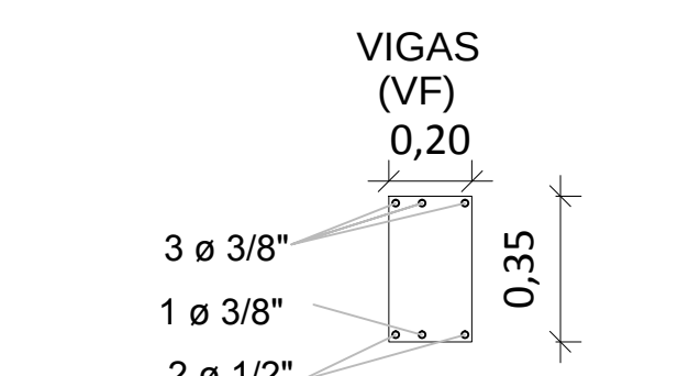
VIGAS (VF) 0,20 0,35 3 \varnothing 3/8" 1 \varnothing 3/8" 2 \varnothing 1/2" Estribos \varnothing 5 c/ 12cm DETALHE VIGA DE FUNDAÇÃO ESCALA 1:20
