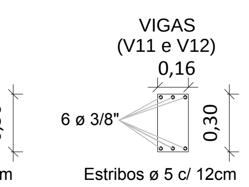
VIGAS (V11 e V12) 0,16 0,30 6 \varnothing 3/8" Estribos \varnothing 5 c/ 12cm DETALHE VIGA ESCALA 1:20
