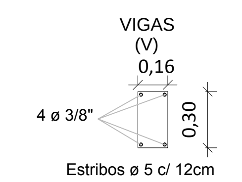
VIGAS (V) 0,16 0,30 4 \varnothing 3/8" Estribos \varnothing 5 c/ 12cm DETALHE VIGA ESCALA 1:20
