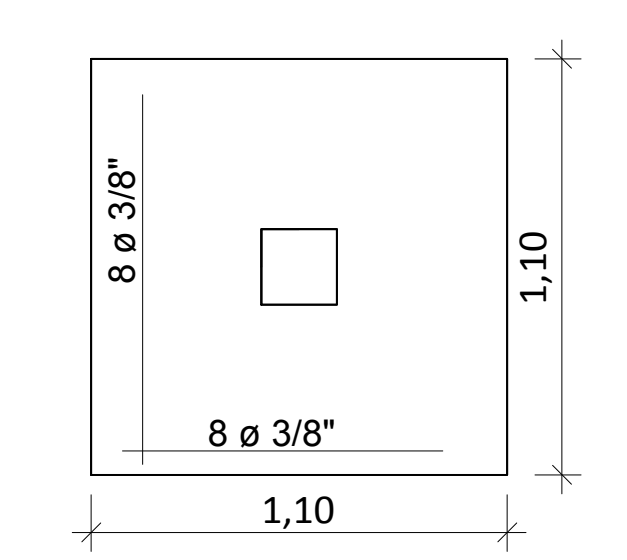
VISTA SUPERIOR DETALHE SAPATA ESCALA 1:20
