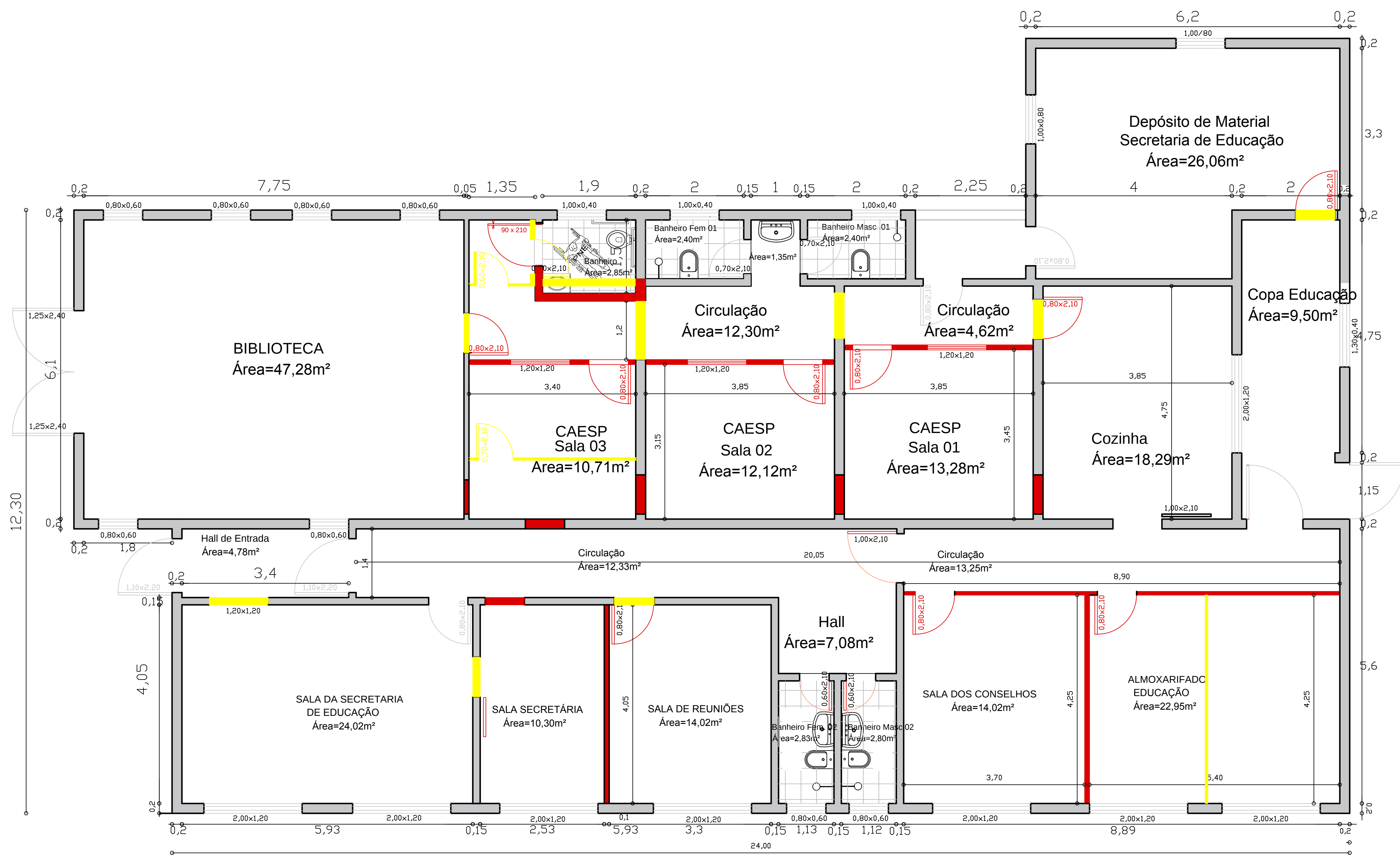
Planta Demolição/construção
