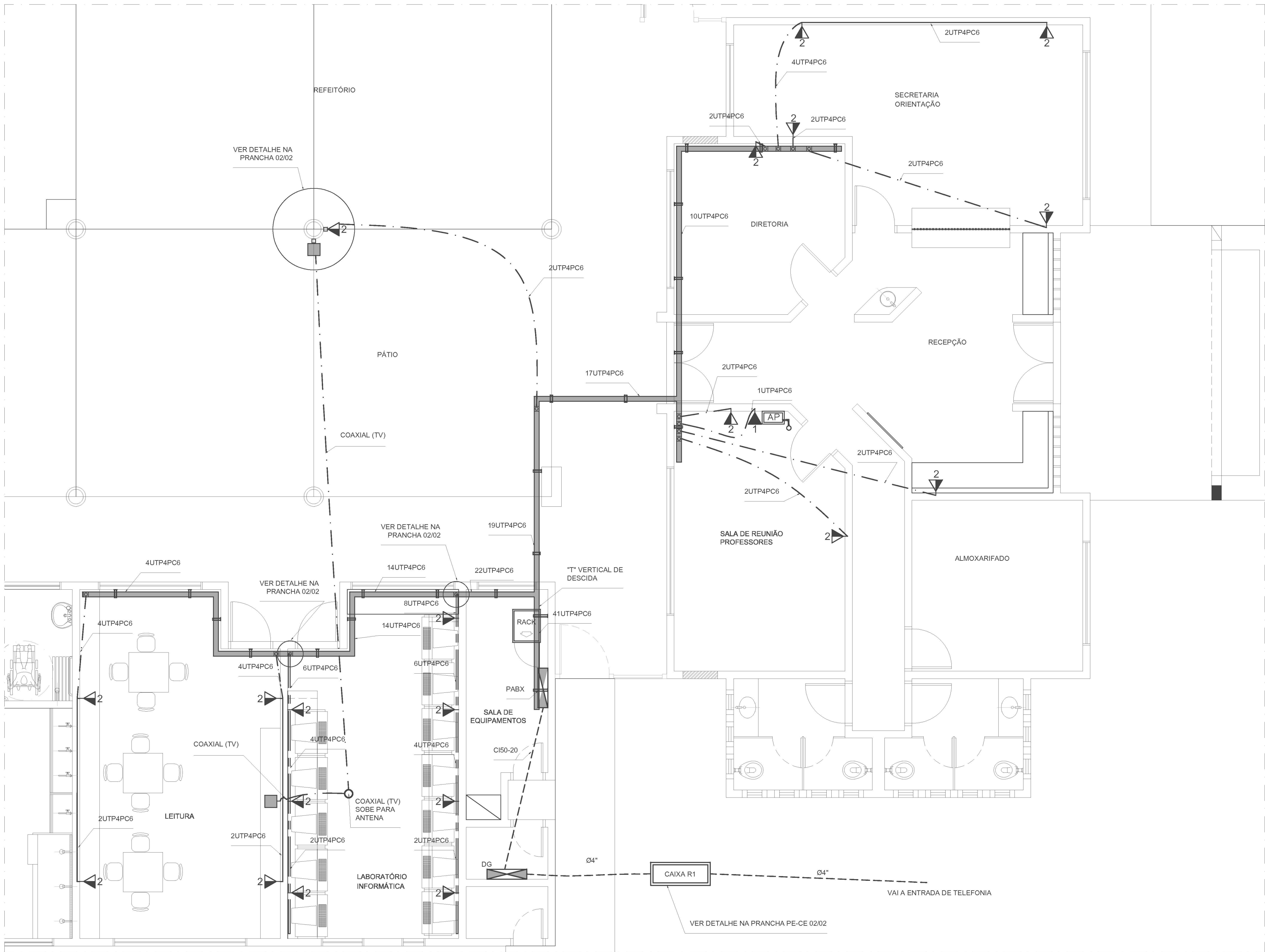
REDE DE CABEAMENTO ESTRUTURADO E ANTENA DE TV PAVIMENTO TÉRREO ESCALA: 1:50
